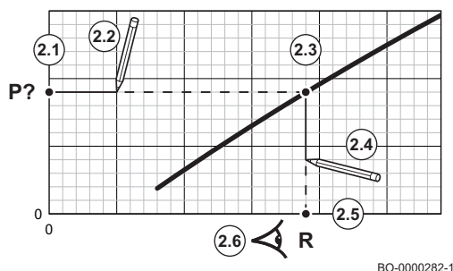
Obr.51 Požadovaný výkon
