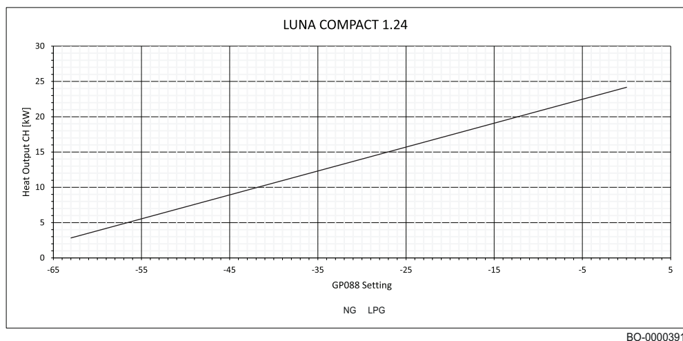
Obr.52 Graf pro LUNA COMPACT – 1.24
