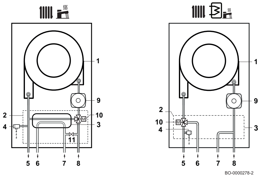
Obr.15 Schematický nákres
