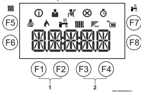
Obr.2 Ovládací panel
