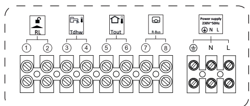
Obr.100 Pripojenia dosky kotla
