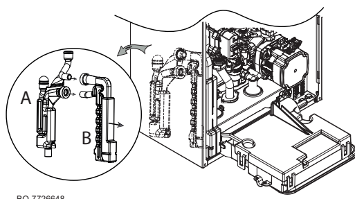
Obr.59 Demontáž sifonu
