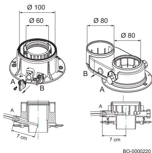
Obr.45 Typ připojení – měřicí přípojka pro spaliny
