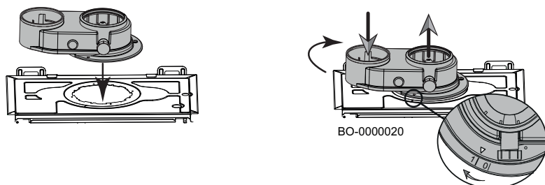
Obr.95 Inštalácia potrubia pri oddelených potrubiach
