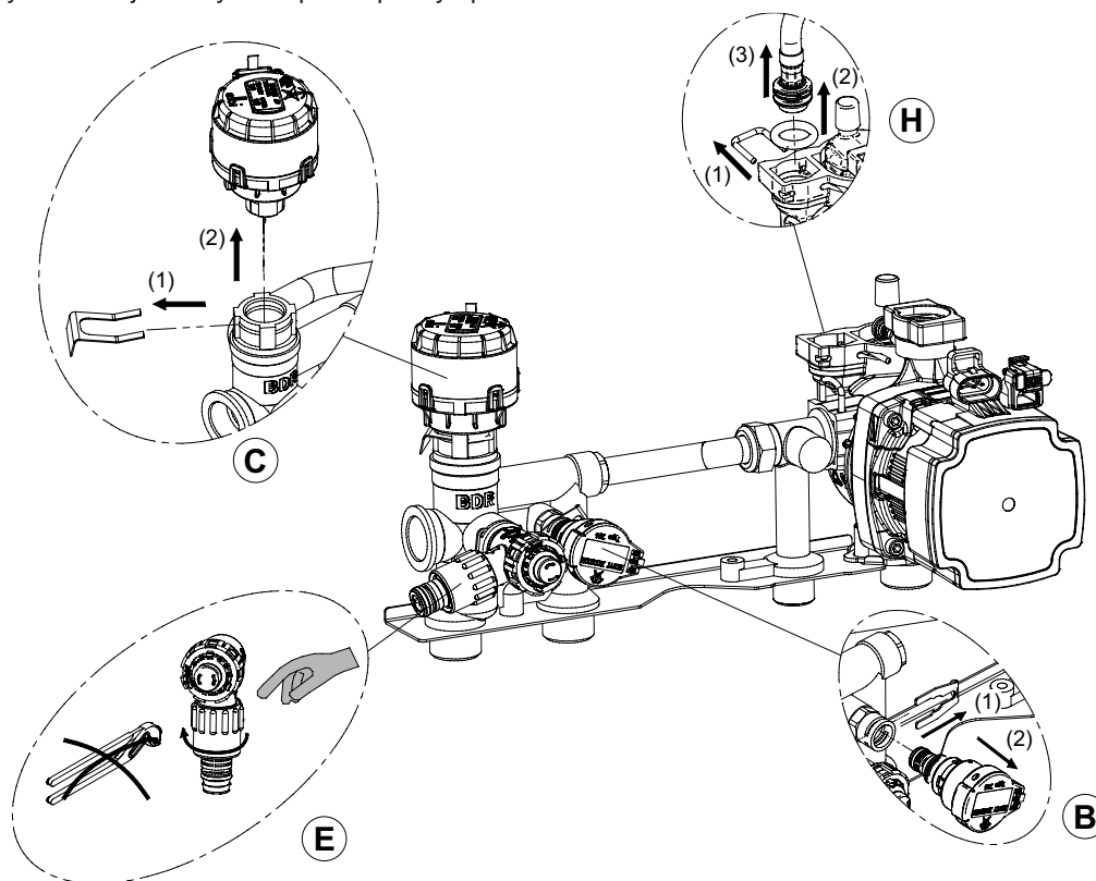
Obr.62 Části hydraulické jednotky kotle pouze pro vytápění
