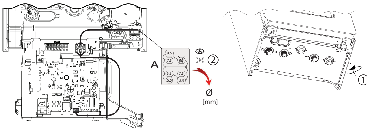
Obr.37 Přidání vodičů ke kotli
