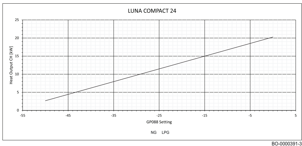
Obr.55 Graf pro LUNA COMPACT – 24
