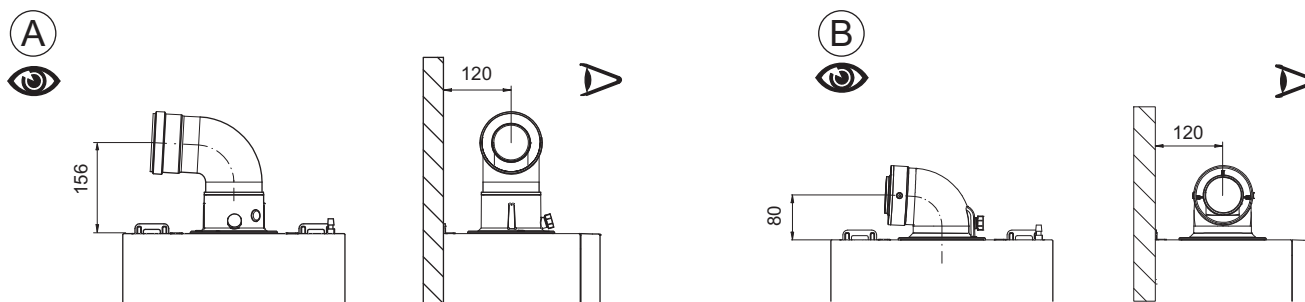
Obr.29 Typ koaxiálního sání – odvodu spalín
