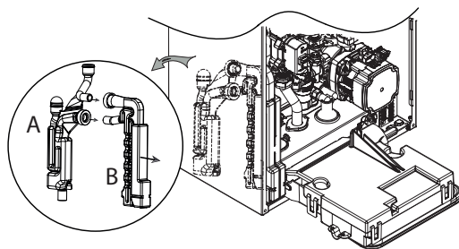
Obr.121 Demontáž sifónu
