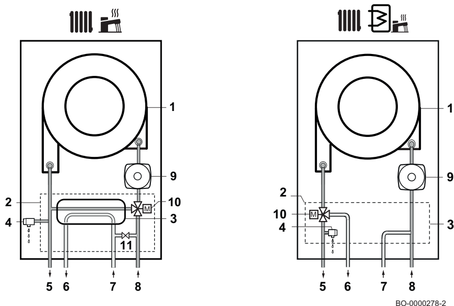
Obr.77 Schematický diagram
