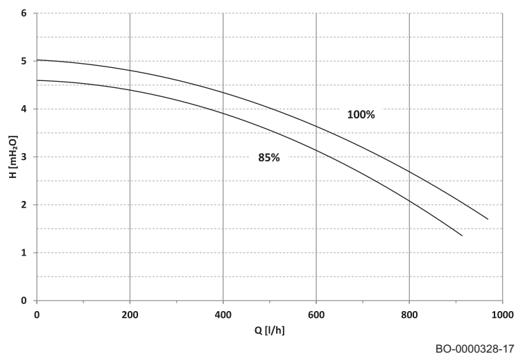
Obr.18 Graf ukazující zbytkové teplo čerpadla na základě průtoku vody
