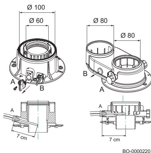
Obr.107 Typy prípojok – merací bod spalín
