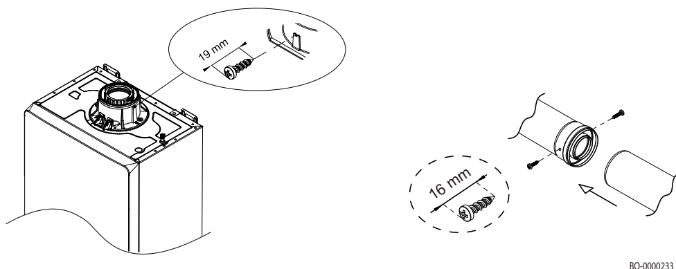
Obr.92 Upevnenie koaxiálneho odvodu spalín
