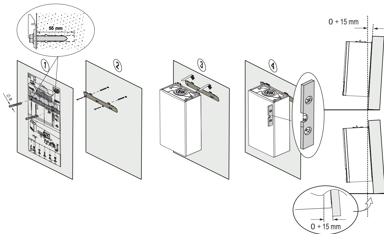
Obr.23 Instalace na stěnu
