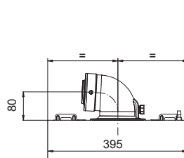
pohľad spredu
