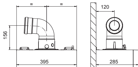
pohľad spredu
