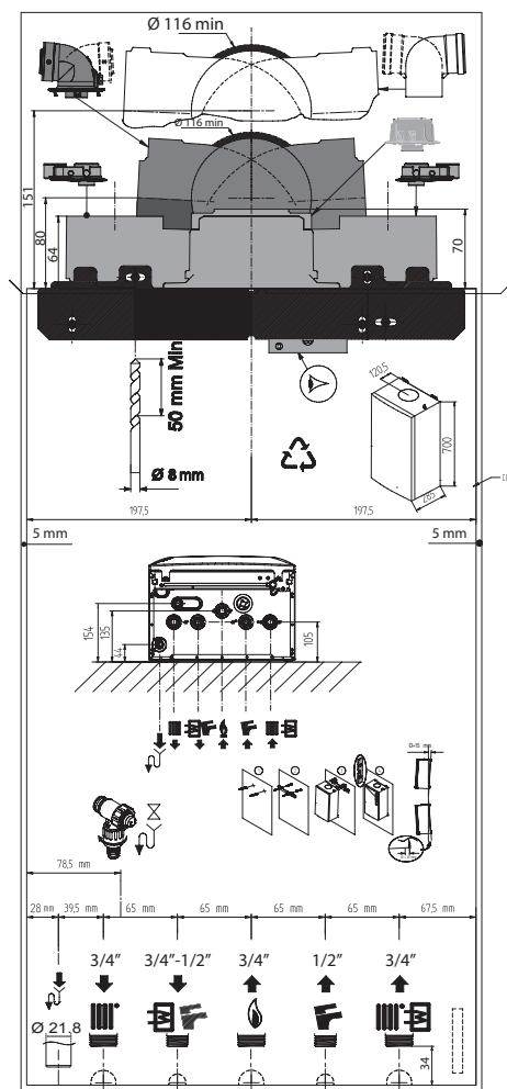
Montážna šablóna
