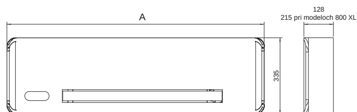
Čelný pohľad
