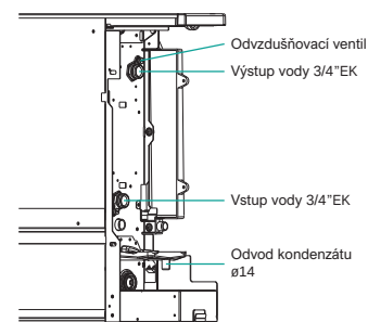
Hydraulické pripojky
